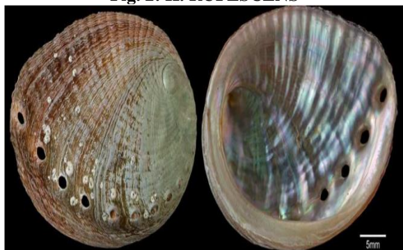
Fig. 3: H. GIGANTEAN
